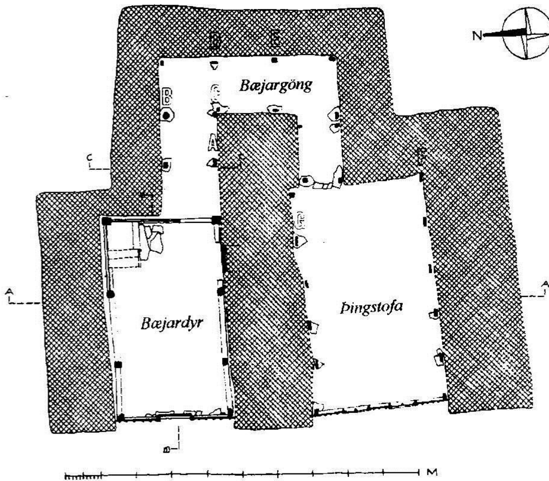
Stóru-Akrar, grunnmynd og útlit. Teikningar Harðar Ágústssonar.
